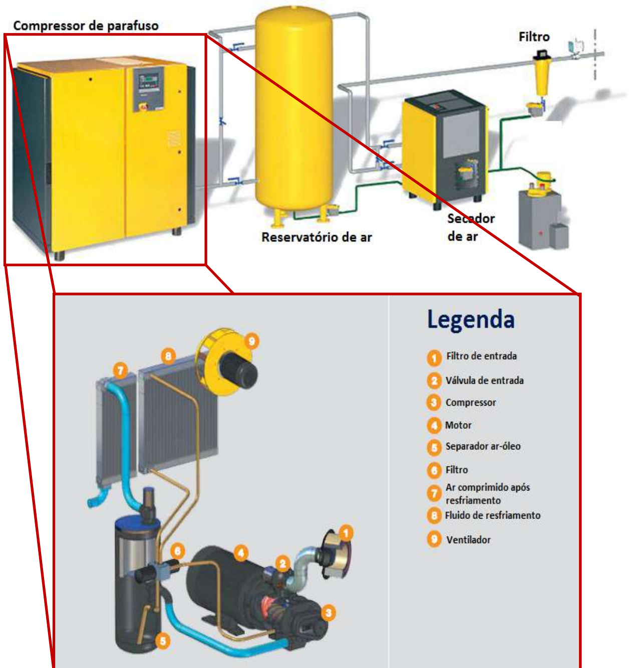
Figura 11 – Componentes internos do compressor de parafuso estacionário
